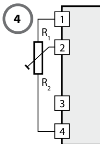
Potenciômetro: 3 fios
