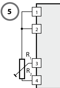
Potenciômetro: 4 fios
