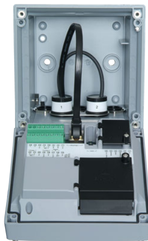
2 Y cable in Stratos Multi E461N
